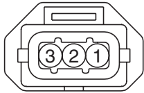
AMP_JPT_03F_B_BSH3
