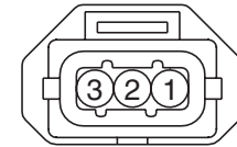
AMP_JPT_03F_B_BSH3
